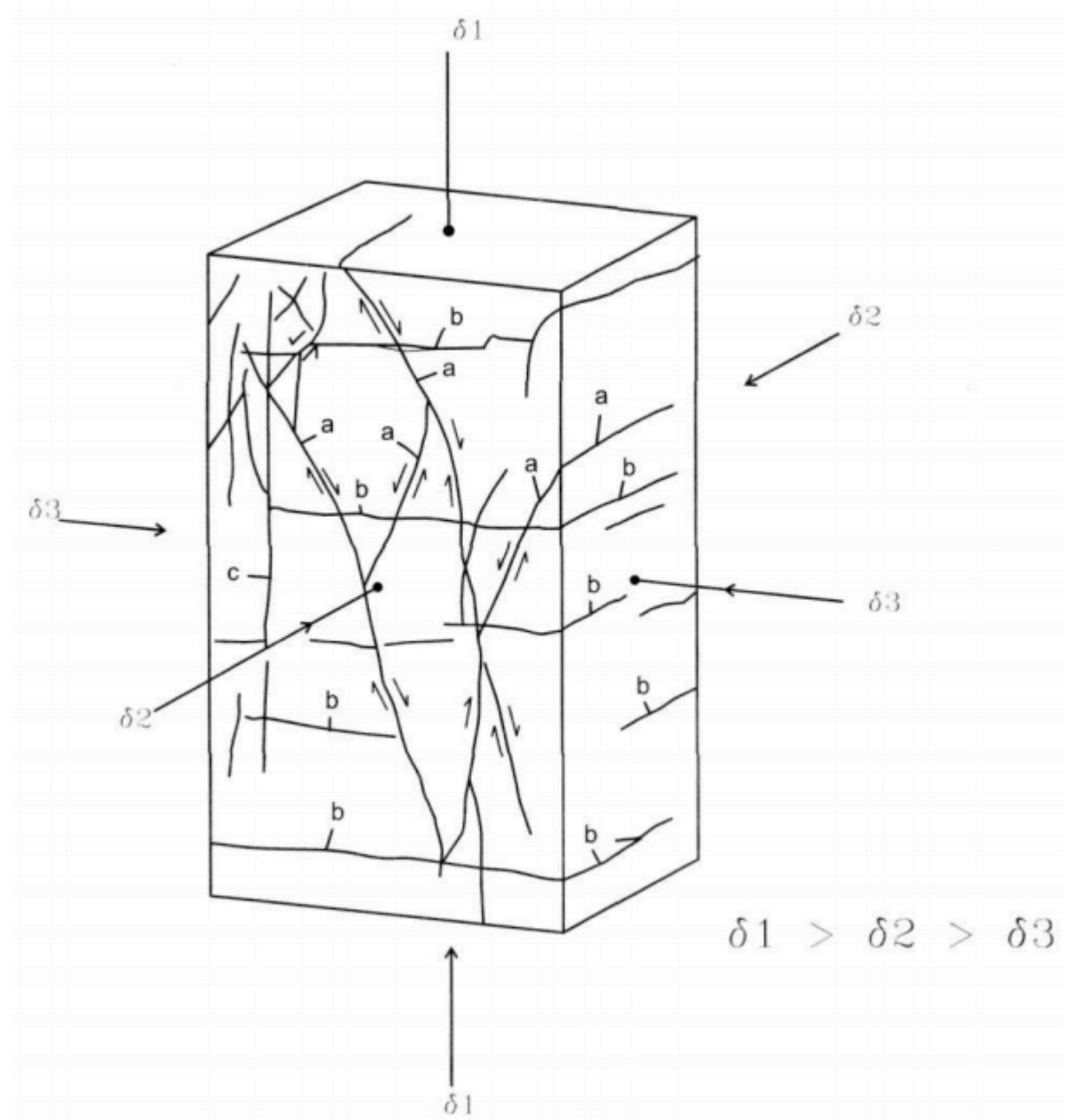
Figura A - Bloque de roca en ensayo de esfuerzos. Tres fuerzas compresivas afectan el bloque: \sigma_1 (1), mayor que \sigma_2 (2), mayor que \sigma_3 (3).
